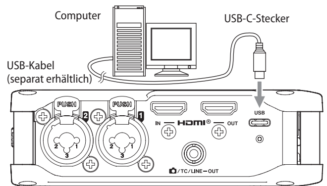
Linke Geräteseite
