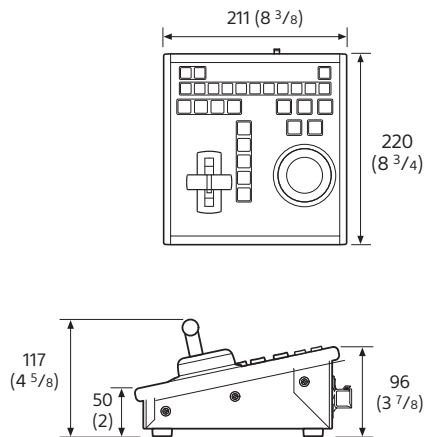
PWSK-4403
